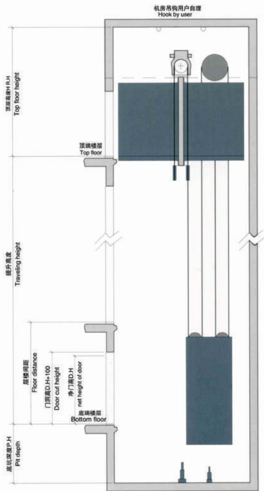
井道立面图 Hoistway elevation
